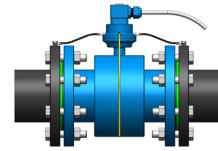
Conductive (metal) pipe
